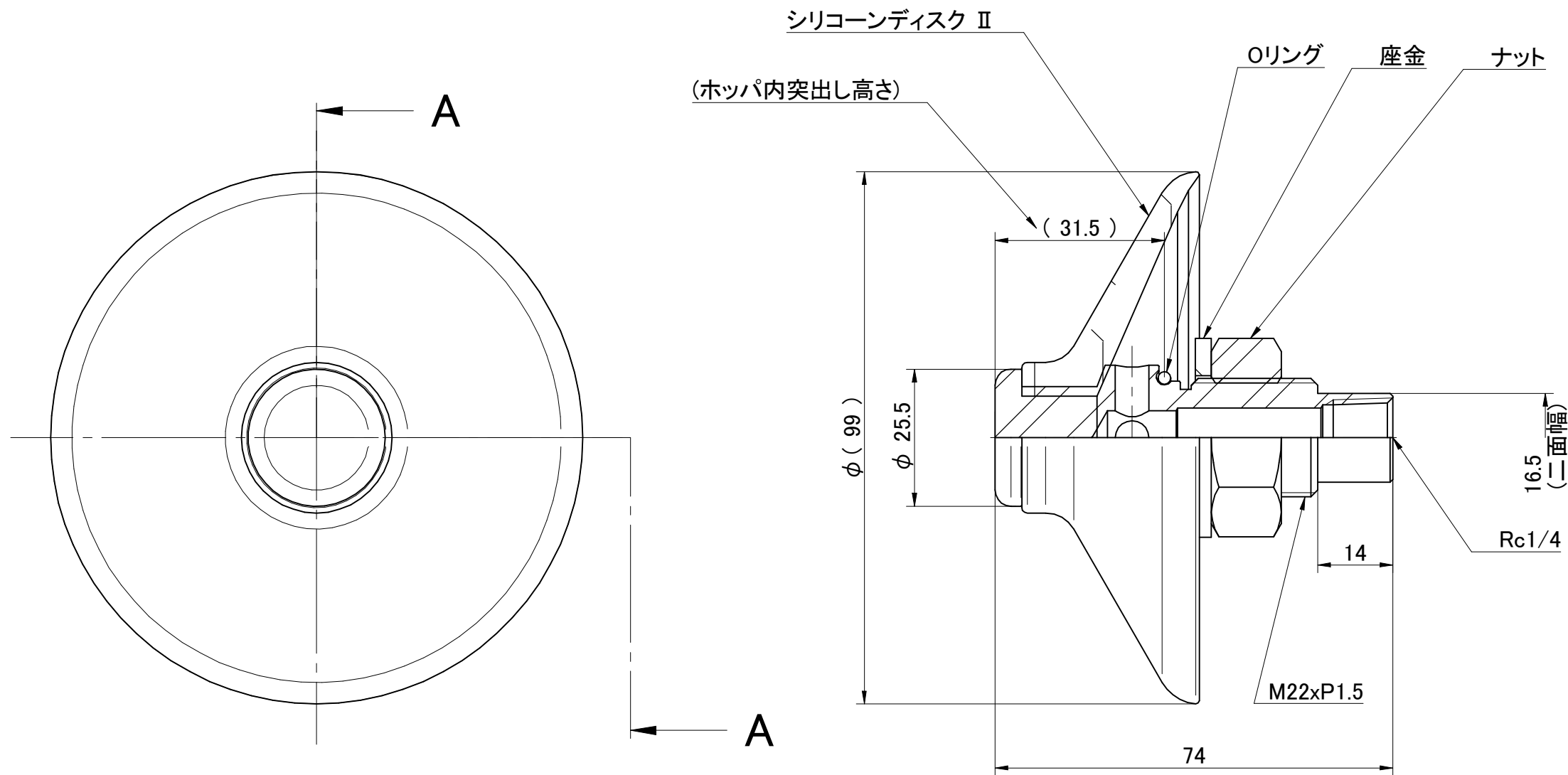
断面 A-A
